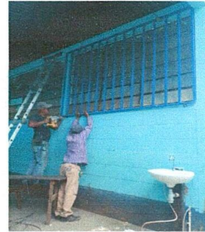
Foto 2: Instalación de balcones de metal
