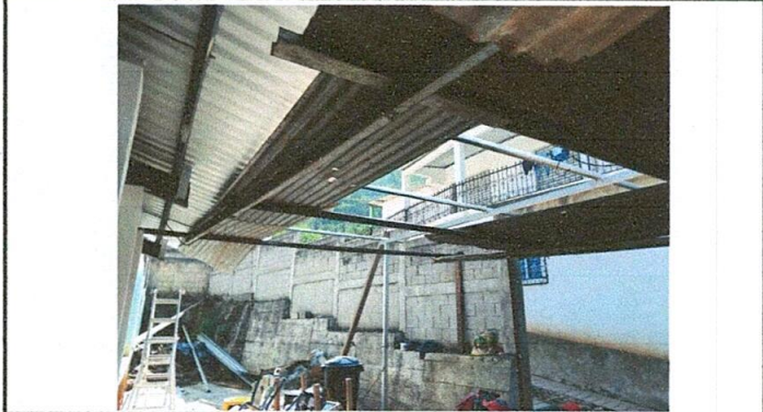
Foto 1: Cubierta de lámina: sustitución de lámina troquelada aluzinc calibre 26 y estructura de techo
