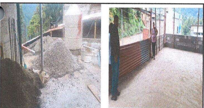
Foto 5: SUSTITUCION DE PARED DE LAMINA POR PARED DE BLOCK
