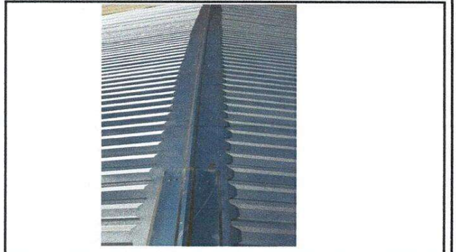
Foto 2: Capotes nuevos colocados
