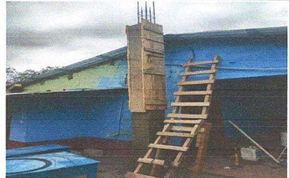
Foto 4: Reforzamiento de la base del tinaco
