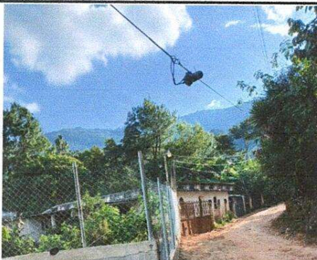
Foto 9: sustitucion de muro perimetral de blok con tubo HG maya galvanizada, soleras intermedias y columnas
