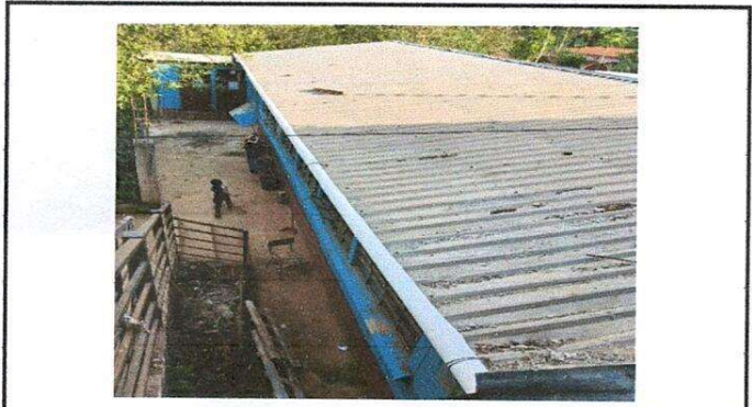
Foto 3: sustitucion de canal por tubo PVC
