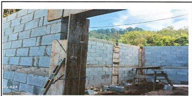
Foto 6: Reparación de muro perimetral de Block (en cocina)
