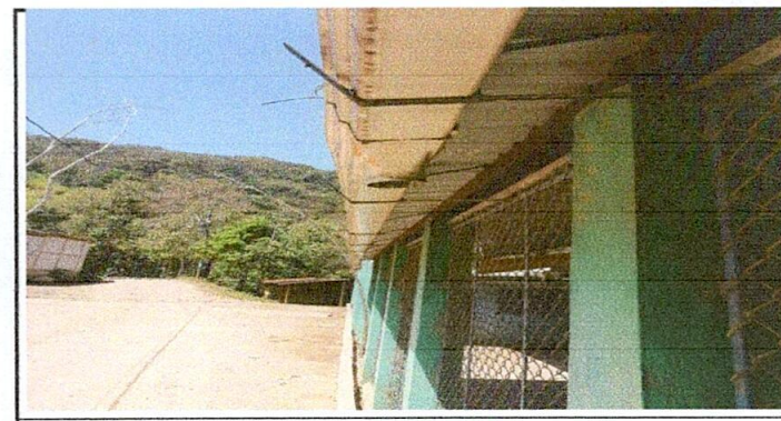
Foto 6: Reparación de bajada de agua pluvial, tubo pvc 3''
