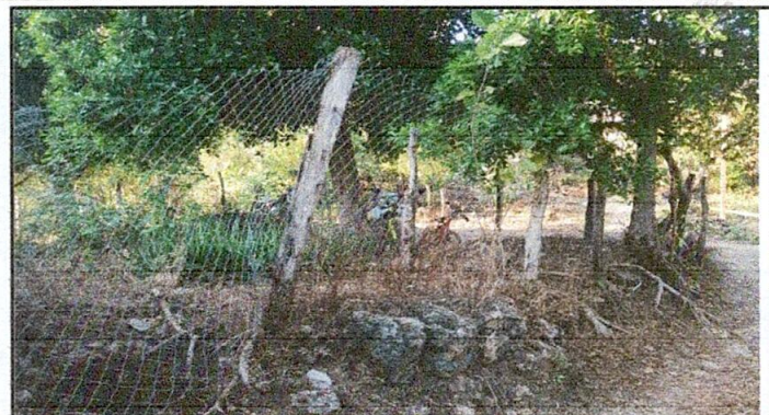
Foto 2: Reparación de muro perimetral de block de 5 hiladas con tubo hg y malla galvanizada (Circulación lateral izquierda del establecimiento)
