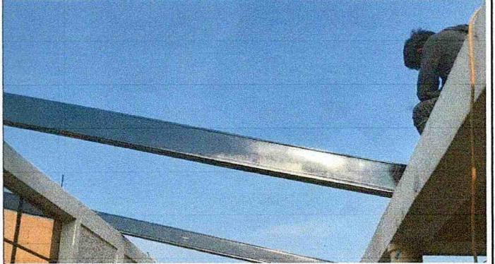
Foto 2: se sustituye la estructura de soporte inicial por vigas de metal.
