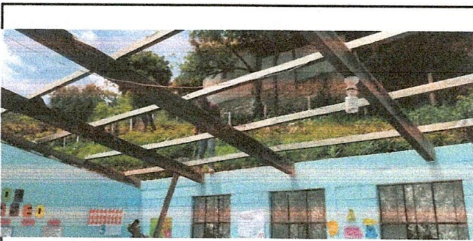
Foto 3: Sustitución de soporte de techo de madera por costaneras galvanizadas
