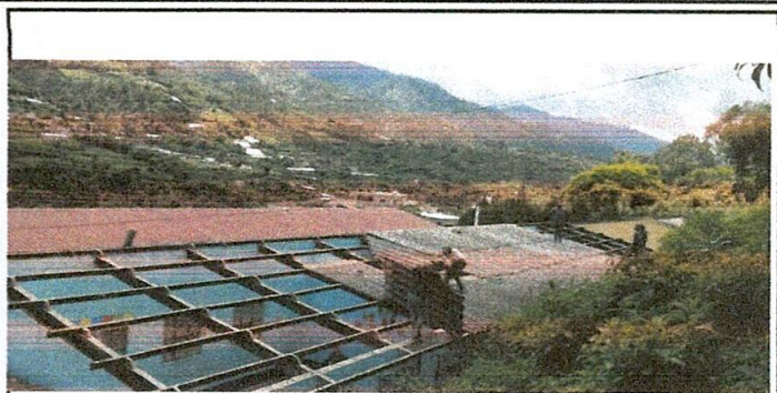
Foto 2: Sustitución de lámina duralita por lámina troquelada
