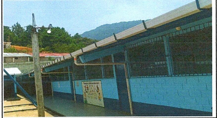
Foto2: renglón finalizado de cambio de canal de metal a PVC
