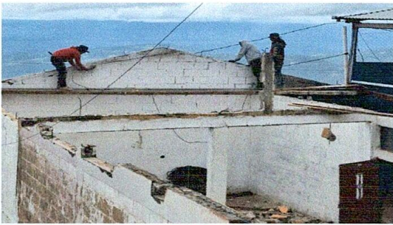
Foto 3: inicio para colocar capote
