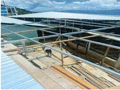
Foto1: Sustitucion de capote en cocina
