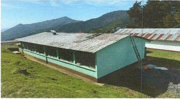
Foto 1: Sustitución de lamina troquelada por lamina troquelada e implementación de canal de metal para captación de aguas pluviales con rotoplas de 2,500 litros
