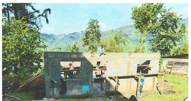
Foto 4: sustitución de paredes de madera por block, sustitución de techo de lamina por techo de lamina con estructura metalica al igual que canal para captación de aguas pluviales y rotoplas de 2,500 litros y colocación
