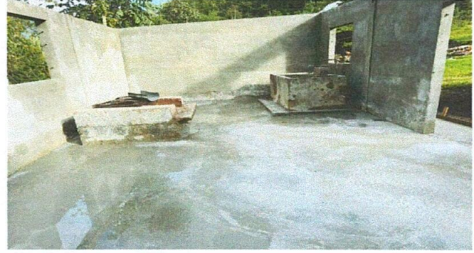
Foto 2: Sustitución de plancha y tubo de chimenea, sustitución de torta de cemento
