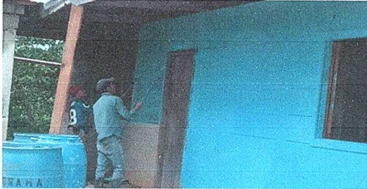
Foto 1: Aplicación de pintura en exterior e interior
