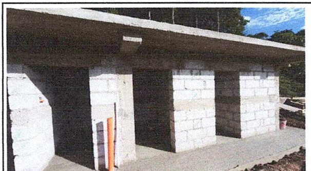
Foto 3. Cada uno de los espacios de los sanitarios ya están terminados, ya sólo falta la instalación de las tazas y puertas.
