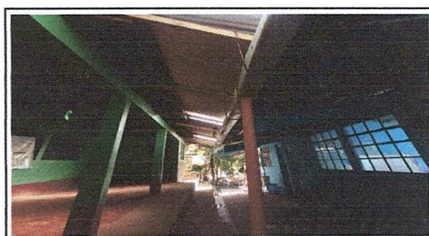
Foto 6. Las láminas troqueladas del techo ya están colocadas en el canal del agua.
