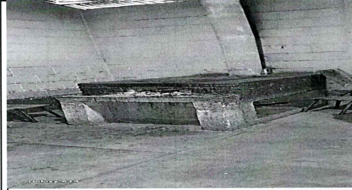
Foto 8 Reparación de cocina: Sustitución Demolición de estufa artesanal existente y al mismo tiempo construir una estufa ecológica, ahorrador de leña (completa), instalación de azulejo de figuras en estufa
