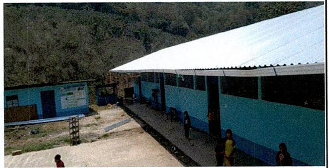
Foto 10 Instalación de canal de pvc y conexión de bajada pluvial
