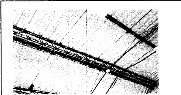
foto 1: Sustitución de lámina, por lámina troquelada aluzinc calibre 26, se filtra el agua y por dentro con pedazos de tabla y pegamento esta tapada
