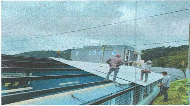
Foto 1: Sustitución de laminas Troqueladas Aluncinc
