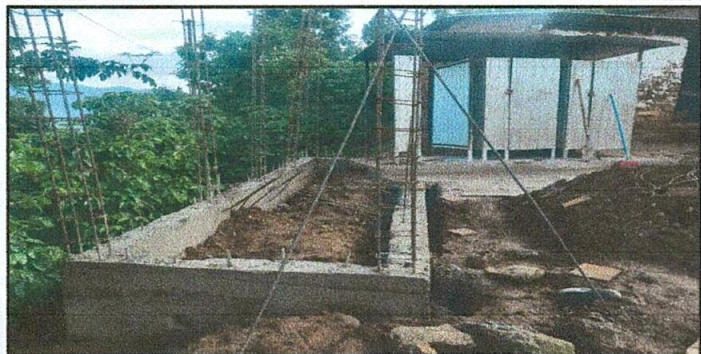
FOTO 1 CIMIENTO DE LOS BAÑOS
