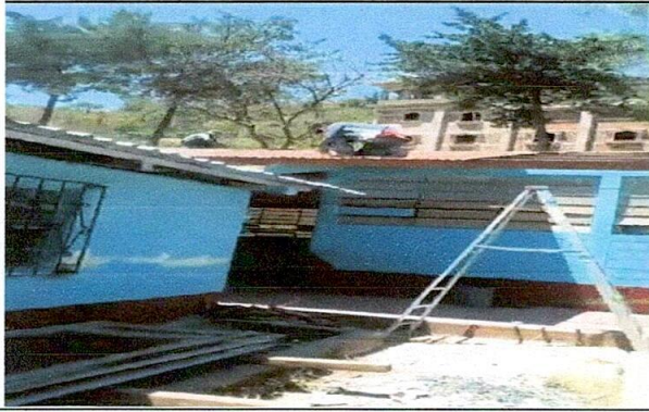
Foto1: Sustitución de lámina simple por lámina troquelada aluzinc calibre 26
