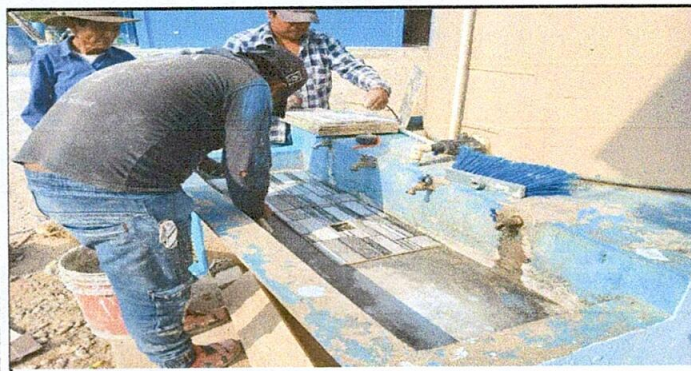
Foto 5: remodelacion de lavamanos
