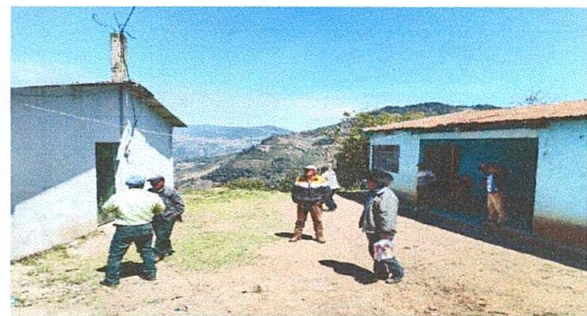
Foto 4: Perspectiva de la escuela donde se ven las láminas oxidadas
