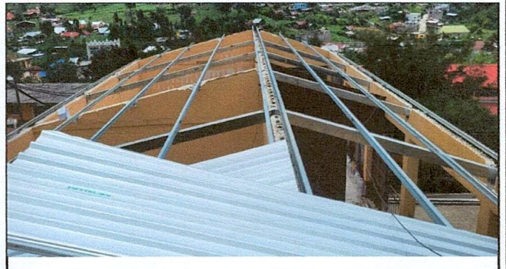
Foto 4. Costaneras instaladas
