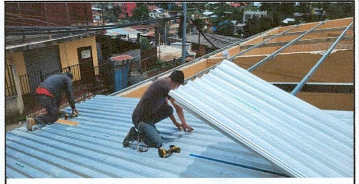
Foto 5. Instalación de láminas
