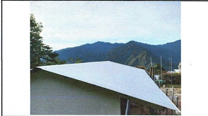
Foto 1: Instalación de lámina troquelada y estructura de techo con satisfacción.
