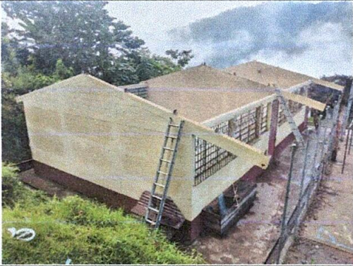
Foto 1: Retirado del techo antiguo para la instalación de nueva estructura.
