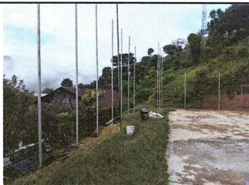
Foto 6: Instalación de tubos galvanizados para el cercado de la cancha polideportiva.
