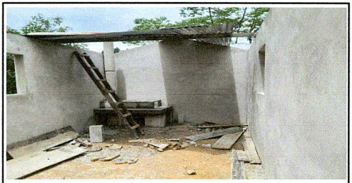
Foto 6: Sustitución de plancha y sustitución de chimenea a concreto. Sustitución de piso a torta de concreto en cocina en proceso.
