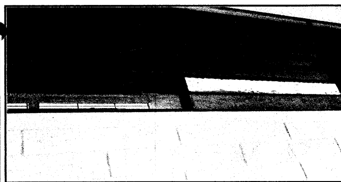
FOTO 5: REPARACIÓN DE PLANCHA DE CONCRETO
