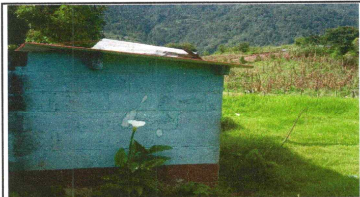
Foto 9: Mejoramiento de pared de block
