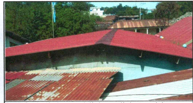
Foto 6: Sustitución de capote de lámina para lámina troquelada
