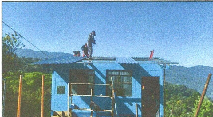
Foto 2: Sustitución de lámina, por lámina troquelada aluzinc
