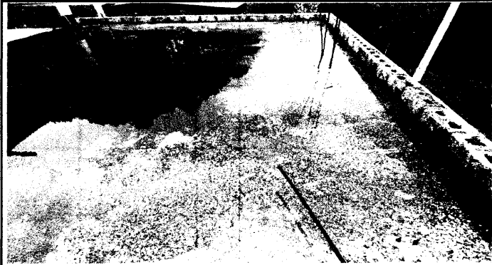
Foto 1: impermeabilización de losa de la Escuela ya está en malas condiciones en la época de lluvia hay bastante humedad, por lo que se prioriza su reparación.
