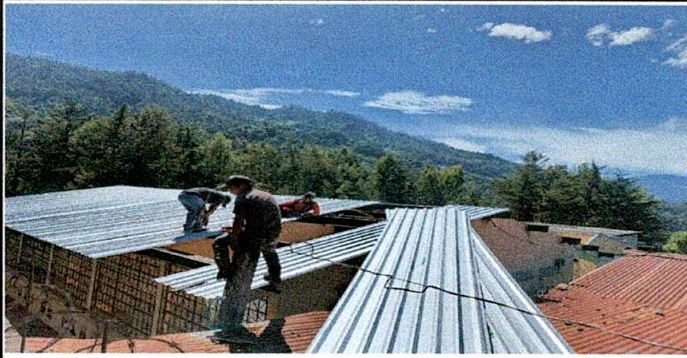
Foto1: Sustitucion de lamina por lamina toquelada
