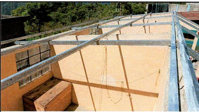
Foto 3: Sustitución de techo de madera por metal
