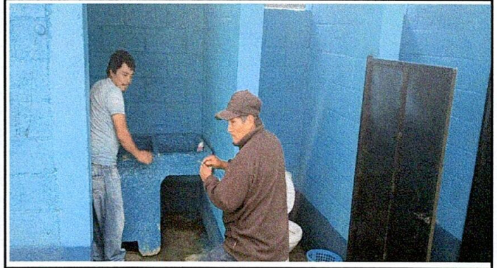
Foto 8: Instalación de pila de cemento de dos lavaderos
