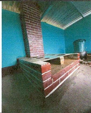
Foto. No. 03. Trabajo terminado en la sustitución de estufa rural de la EORM, aldea Xocol.
