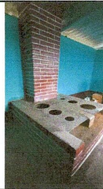
Foto. No. 04. Trabajo terminado en la sustitución de estufa rural de la EORM, aldea Xocol.
