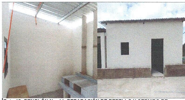
Foto 12: RENGLÓN No. 11. REPARACIÓN DE REPELLO Y CERNIDO DE PAREDES, Mejoramiento repello en pared (Repello de interior y exterior de la cocina)
