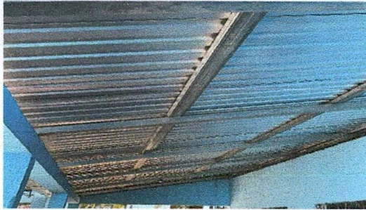
Foto 1: Láminas y madera en malas condiciones.
