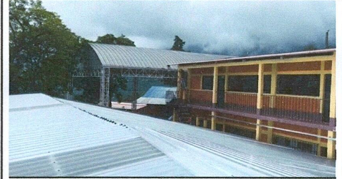
Instalación de Láminas y costaneras Módulos 1 al 3
