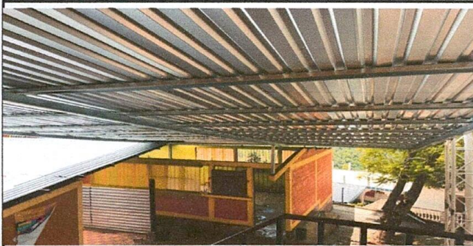
Sustitución de costaneras en Módulos 1, 3 y 4
