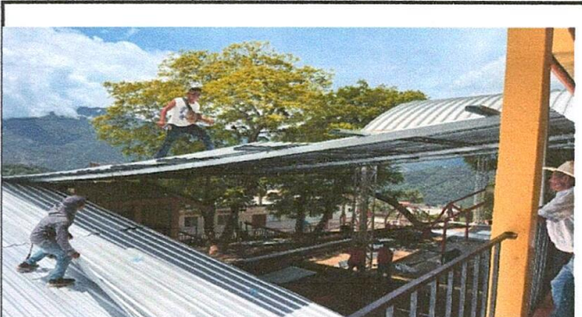
Módulo 4 con láminas y costaneras colocadas
