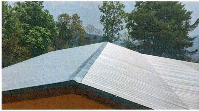
Foto 1: Sustitución de lámina y capotes calibre 26 en aulas y patio.
