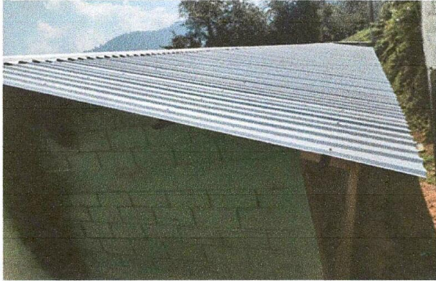
Foto 1: Se realizó sustitución de lámina por lámina troquelada aluzinc calibre 26, debido a que en invierno caían muchas goteras sobre los escritorios y muebles del aula.
