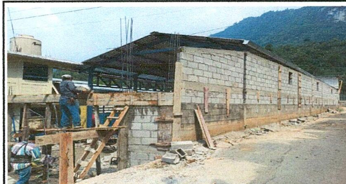
Foto 6: REPARACIÓN DEL MURO DE CONTENCIÓN
