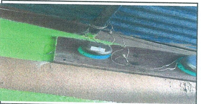
Foto 5: el cableado es deficiente porque tiene varias reparaciones y no funciona adecuadamente, por esa razon se queman constantemente los focos y aparatos electricos.
