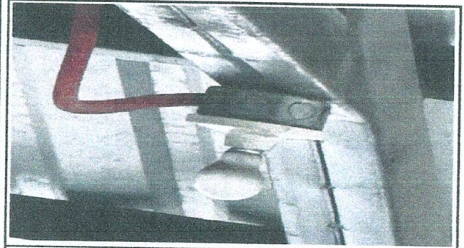
Foto 3: Relaciondo a la instlación electrica en general está en mal estado porque tiene corte circuito porque los cable estan deteriorados y topan con el metal, los focos no son adecuados para la cancha ni para las aulas.
