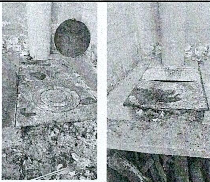
Foto 5: reparación de estufa, cambiando planchas y tubo de salida de humo y ladrillos.
