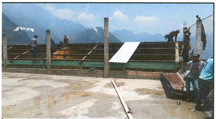
Foto 4: Colocando lámina troquelada en los 2 aulas y así nos evitamos las goteras generadas por las lluvias durante el invierno.
