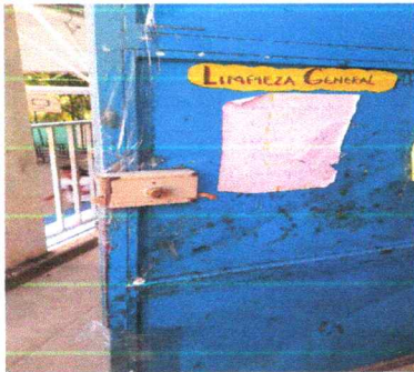
Foto 15: PUERTAS DE METAL, SUSTITUCION DE CHAPAS
