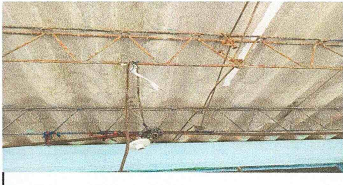
Foto 4: Techo de fibrocemento dañado por lluvias y soporte de metal tipo joist oxidado en mal estado en la mayor parte.
