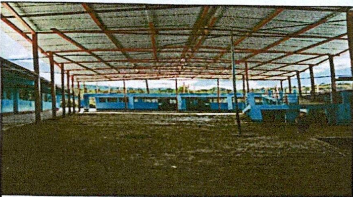
Foto 3: Sustitución de hierro por costanera
