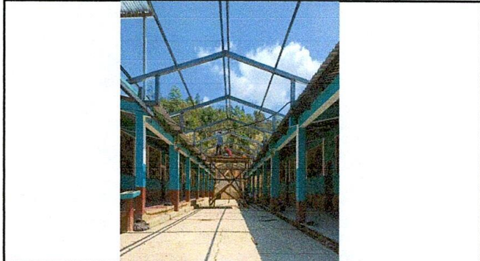
Foto1: Aquí se instalan las primeras tijeras metálicas.
