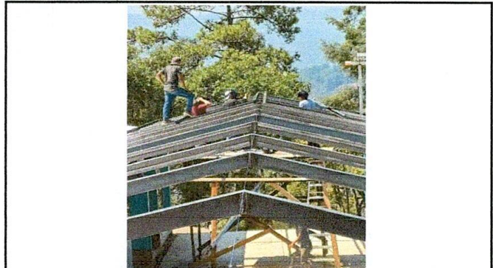
Foto 2: Luego proceden terminan de colocar las tijeras.
