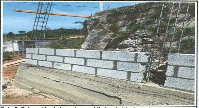
Foto 5: Colocación de las primeras hiladas de block en el muro de contención sobre la fundición de la base de concreto.
