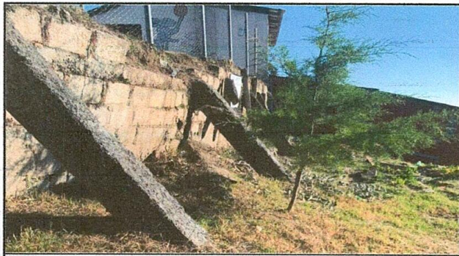
Foto 1: Vista previa del estado del muro de contención de la escuela
