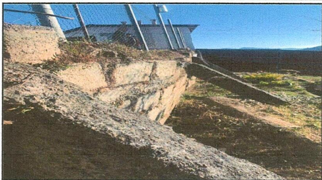
Foto 2: El muro de contención a punto de colapsar, las vigas de concreto lo están deteniendo aún.
