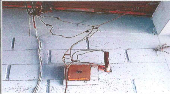
Foto 13: CABLEADO CON CONEXIONES INCORRECTAS
