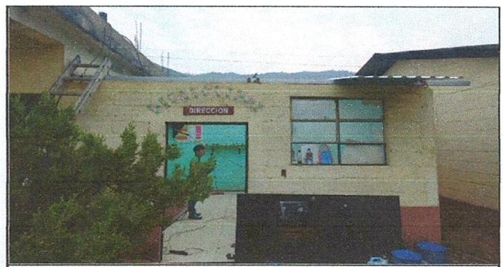
Foto 6: La estructura de madera del techo de la Dirección del establecimiento ha sido removido y se inicia la colocación de la estructura portante de metal; así como la colocación del porcelanato en el
