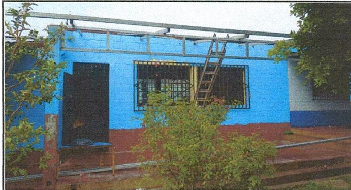
Foto 1: Se observa que las láminas y la estructura del techo del corredor, fueron quitadas y la nueva estructura ya está colocada.
